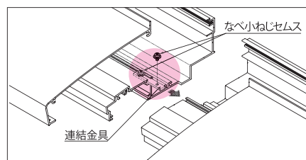
アドビュー連結セット(アドビュー-N2・L2・U共通) カラー:S/シルバー ※連結金具×1ヶ・ネジ・テープのセットです。 ※旧アドビューとアドビュー-N2は連結できません。
