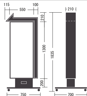
FX-S42LED
