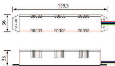
●FDCV0127E1LI
