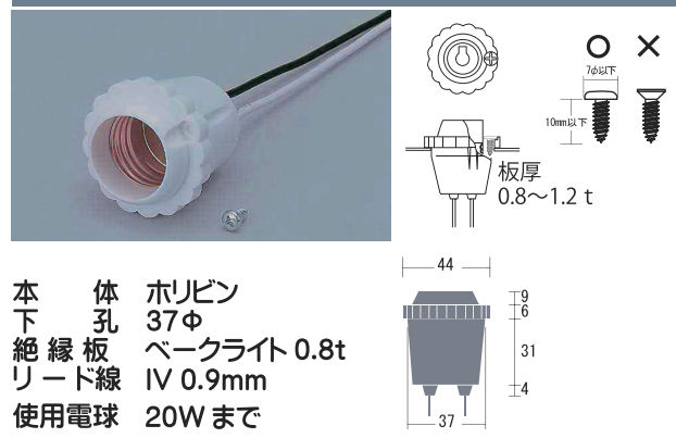
PE-26S 白 ※20個単位での販売になります。
